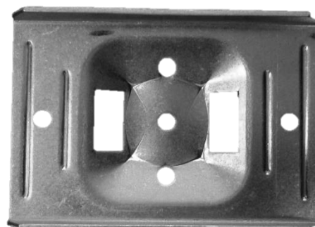
Alu pladeholder til rør: Vare nr. 16032 110 mm. x 70 mm. Alu pladeholder til ujævn underlag Vare nr. 16110 110 mm. X 70 mm.
